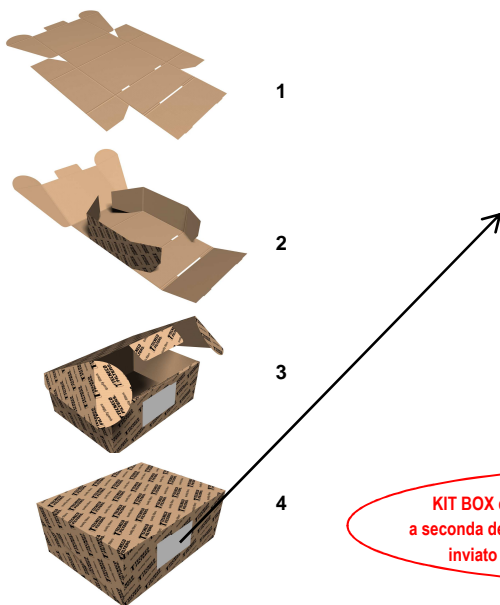
KIT BOX facilmente componibile senza l'uso di nastro adesivo
